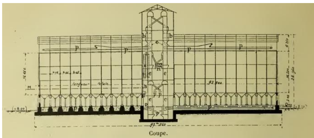
Figura 5: Plano de corte del elevador del puerto de Rosario.
