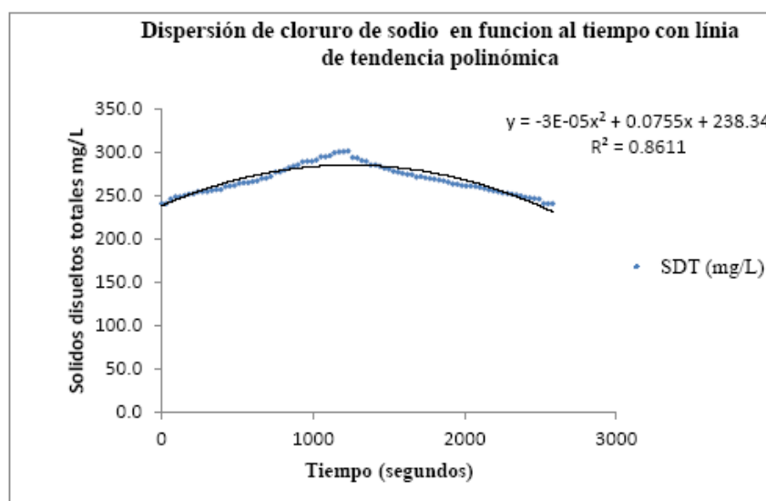
Figura 3. Conductividad eléctrica de las muestras tomadas cada 30 segundos en unidades de sólidos disueltos totales (mg/L) en función del tiempo, y ajuste polinómico.
