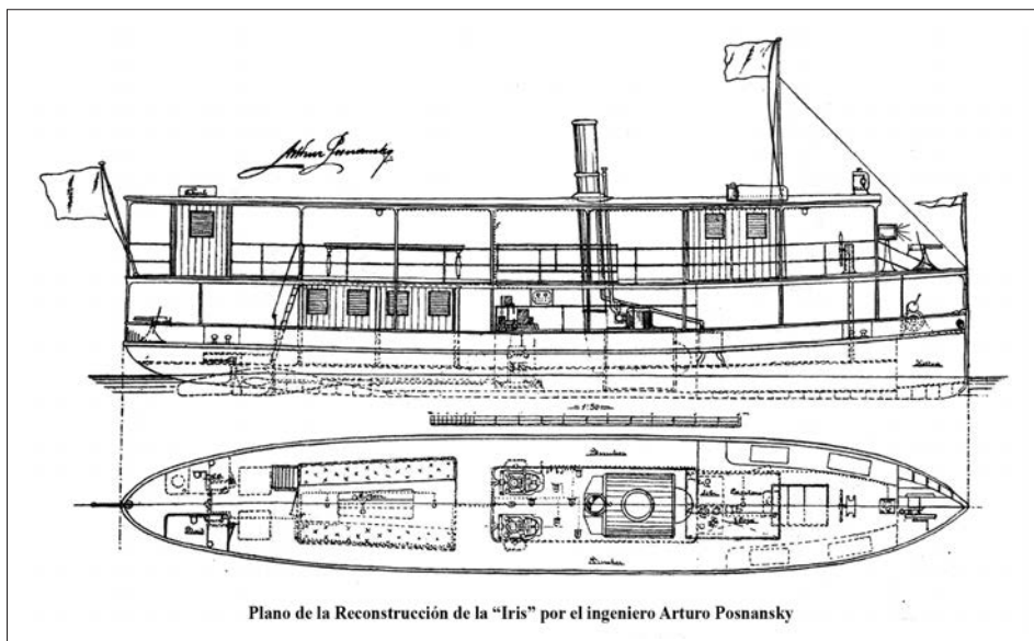
Figura 3. Plano de reconstrucción de la Iris.
